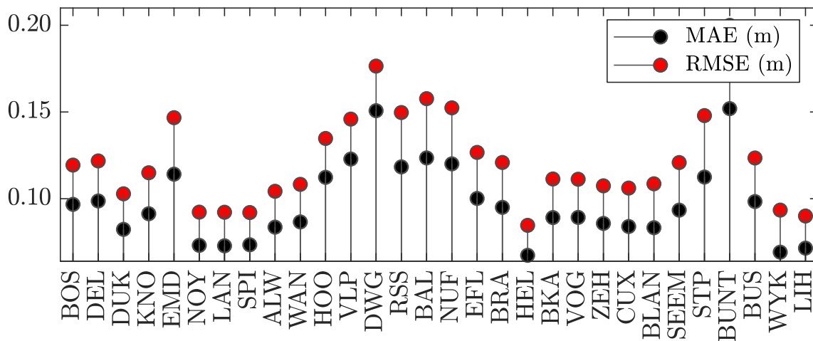
Abbildung 11: mean absolute error (MAE) und root mean square error (RMSE) des Wasserstands im 2002
