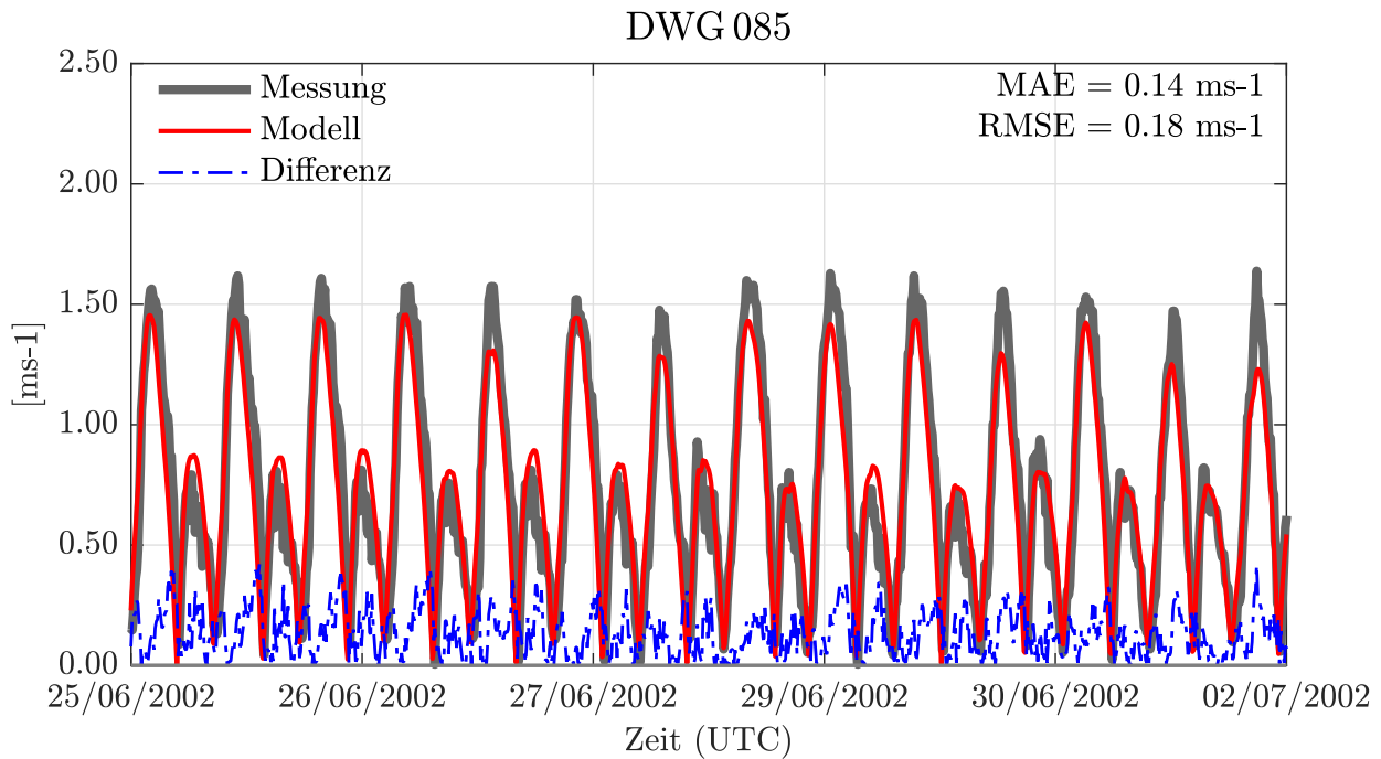
Abbildung 13: Ganglinie der Strömungsgeschwindigkeit (Magnitude) im Jahr 2002 in Dwarsgat mit der Angabe des MAE und des RMSE, den Modelldaten in rot, den Messdaten in grau und den Differenzen in blau.
