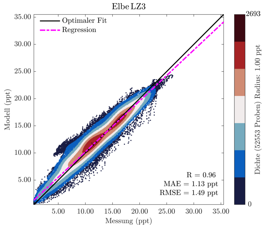
Abbildung 17: Scatterplot des Salzgehalts im Jahr 2002 in LZ3
