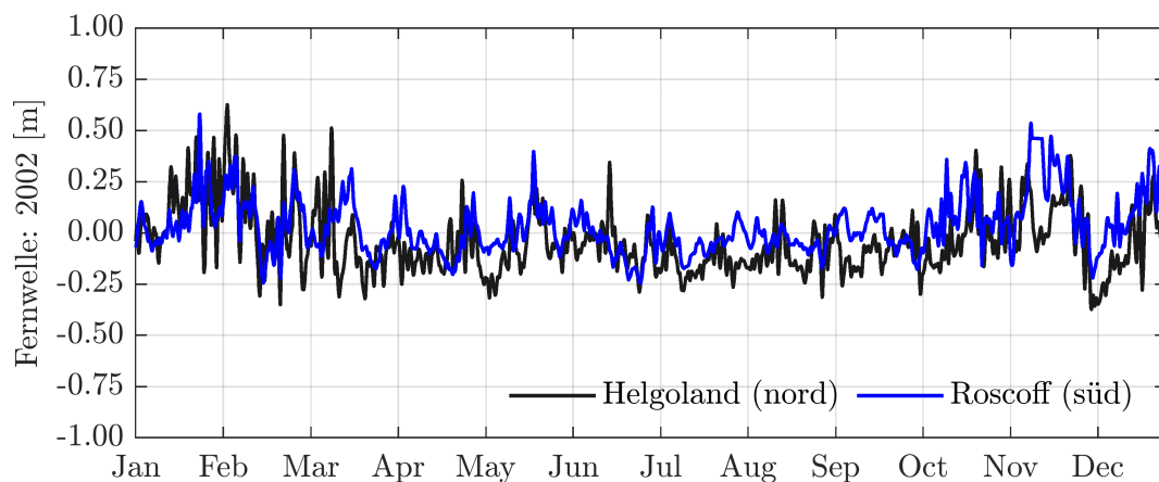
Abbildung 5: Fernwelle am Nord- und Südrand im Jahr 2002
