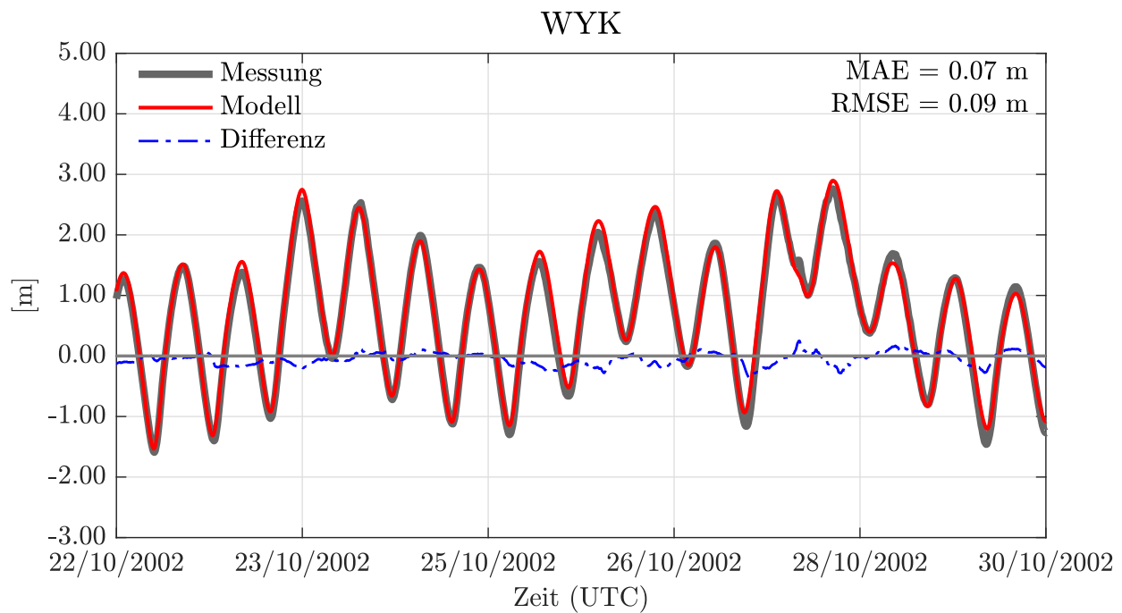
Abbildung 9: Pegelganglinien des Wasserstandes in Wyk (2002) mit der Angabe des MAE und des RMSE, den Modelldaten in rot, den Messdaten in grau und den Differenzen in blau.
