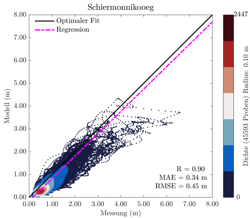
Abbildung 21: Scatterplot der signifikante Wellenhöhe ( h_{sig} ) in Schiermonnikooeg (2002)
