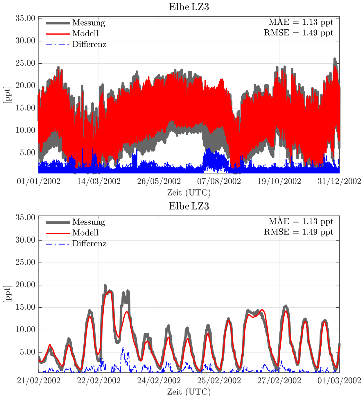
Abbildung 16: Ganglinie des Salzgehalts im Jahr 2002 in LZ3 mit der Angabe des MAE und des RMSE, den Modelldaten in rot, den Messdaten in grau und den Differenzen in blau.
