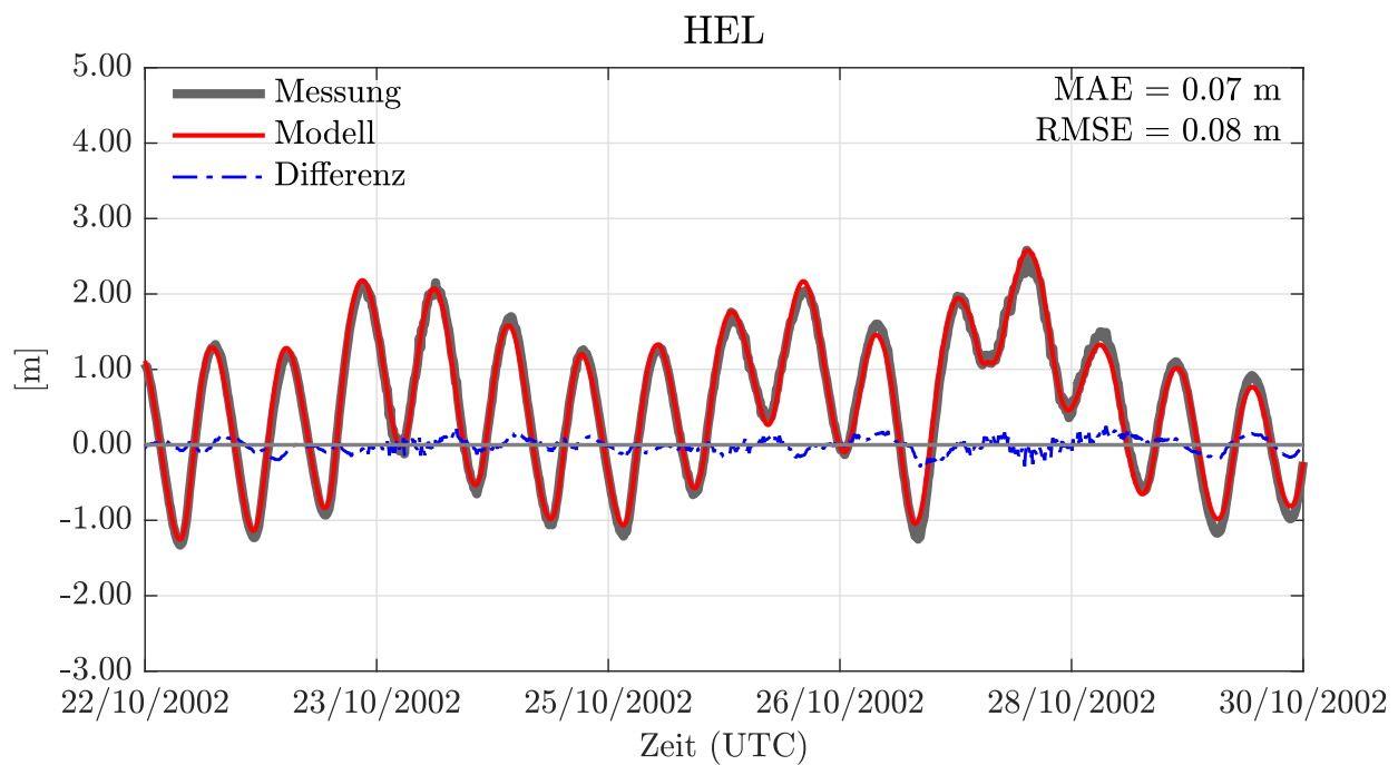
Abbildung 8: Pegelganglinien des Wasserstandes in Helgoland (2002) mit der Angabe des MAE und des RMSE, den Modelldaten in rot, den Messdaten in grau und den Differenzen in blau.
