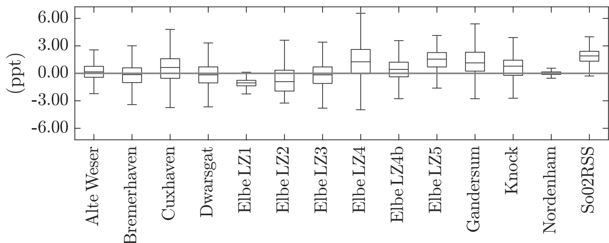
Abbildung 18: Fehlerverteilung des Salzgehalts für das Jahr 2002
