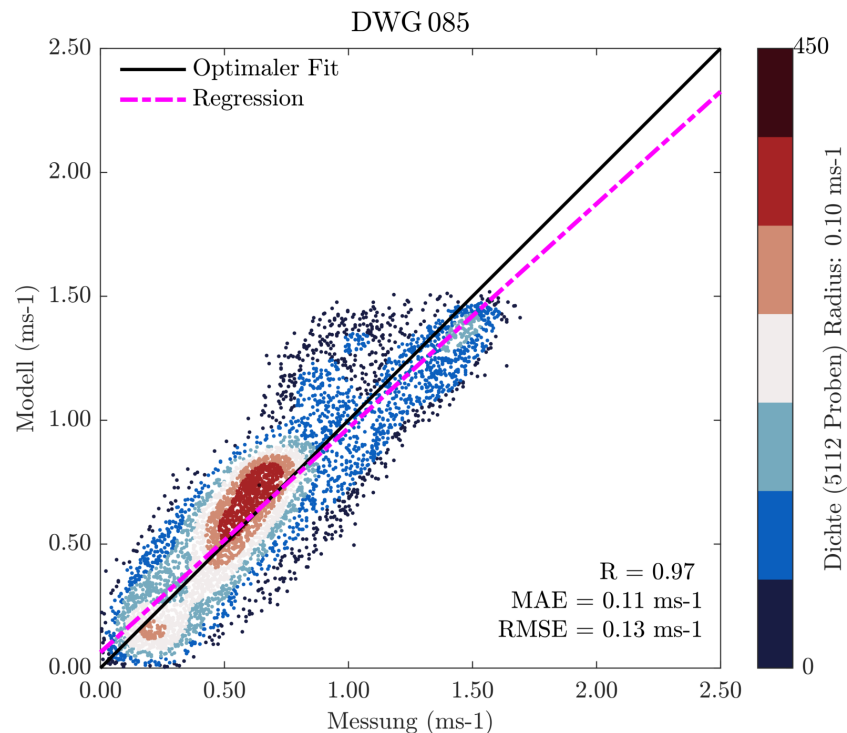
Abbildung 15: Scatterplot der Strömungsgeschwindigkeit (Magnitude) im Jahr 2002 in Dwarsgat
