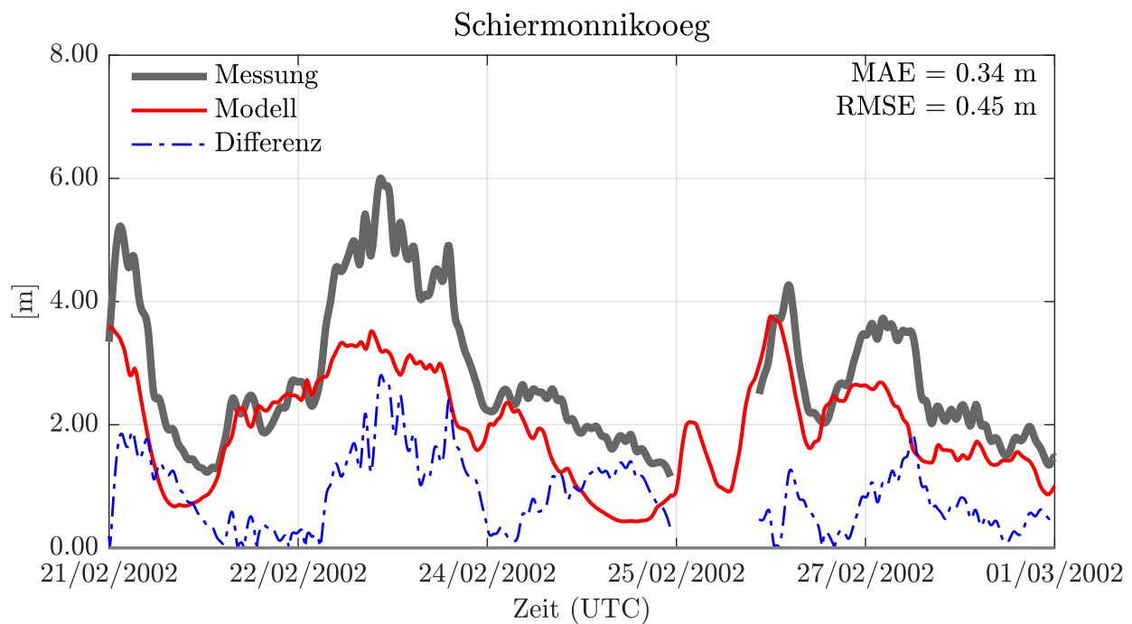
Abbildung 20: Pegelganglinien der signifikante Wellenhöhe ( h_{sig} ) in Schiermonnikooeg (2002) mit der Angabe des MAE und des RMSE, den Modelldaten in rot, den Messdaten in grau und den Differenzen in blau.
