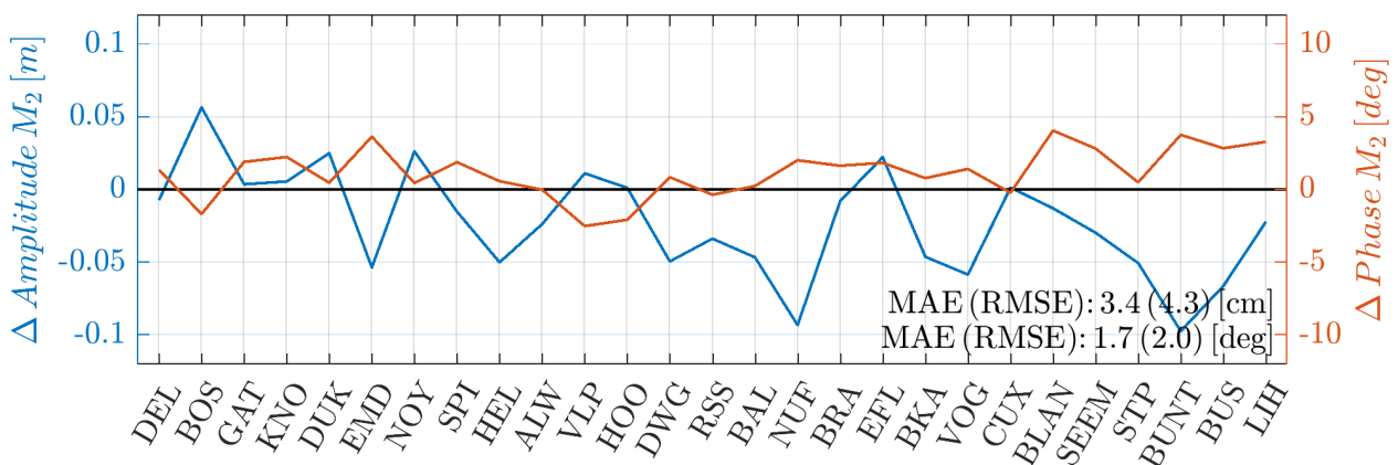
Abbildung 7: Ergebnisse der Partialtidenanalyse aus 2002 als Differenz zwischen Messung und Modell von Amplitude und Phase der M_2 .
