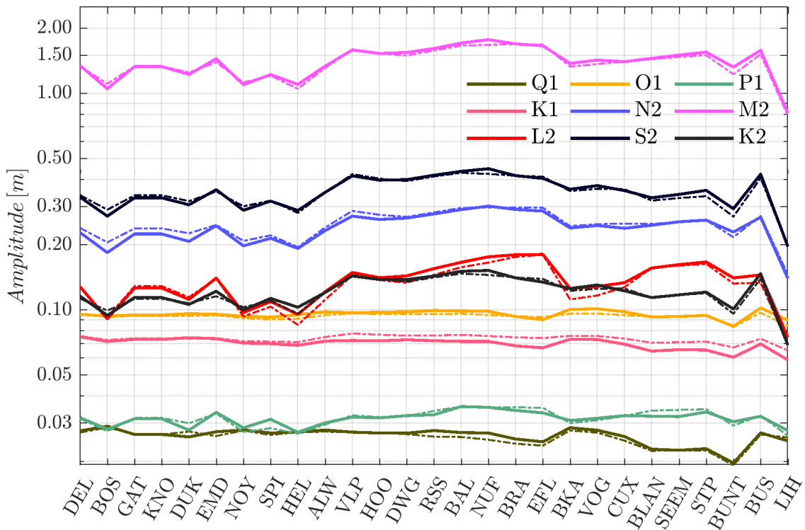
Abbildung 6: Ergebnisse der Partialtidenanalyse aus 2002 für Q1, O1, P1, K1, N2, M2, L2, S2 und K2 für die Deutsche Bucht. Flachwassertiden werden im Jahreskennblatt nicht gezeigt. Durchgezogene Linien repräsentieren die Messung, gestrichelte das Modell.
