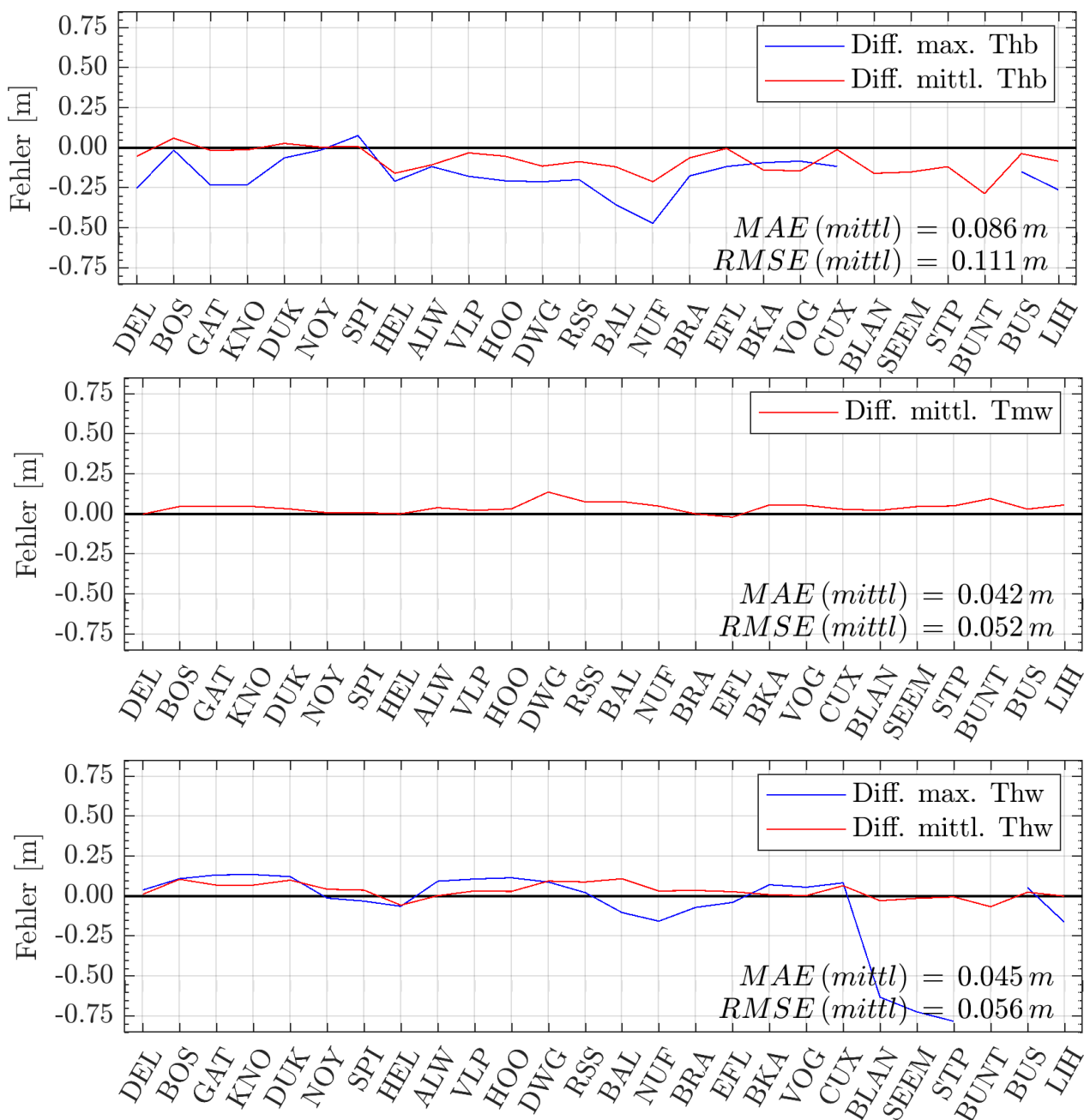
Abbildung 12: Fehler des mittlerer Tidehub (mittl. Thb), mittleres Tidemittelwasser (mittl. Tmw) und mittleres Tidehochwasser (mittl. Thw) im Jahr 2002
