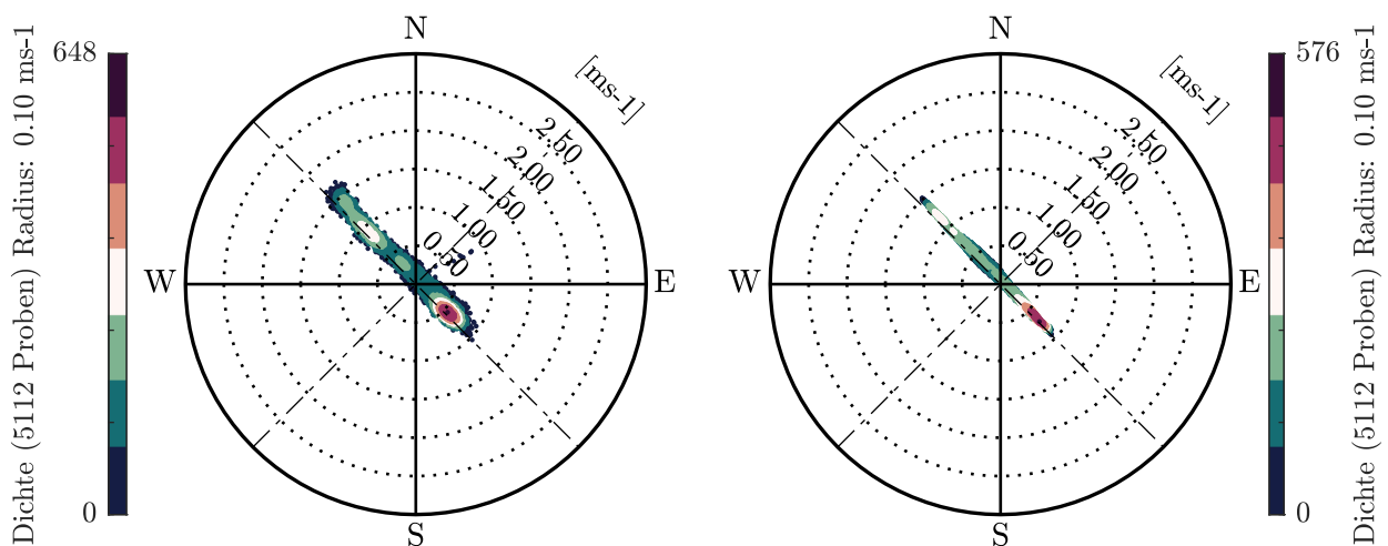
Abbildung 14: Hodograph der Strömung im Jahr 2002 in Dwarsgat, mit einem robusten Regressionsansatz (pinke, gestrichelte Linie)
