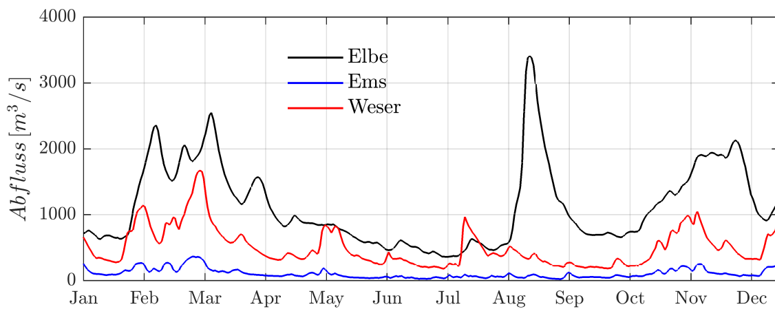
Abbildung 3: Abfluss in Weser, Ems und Elbe im Jahr 2002
