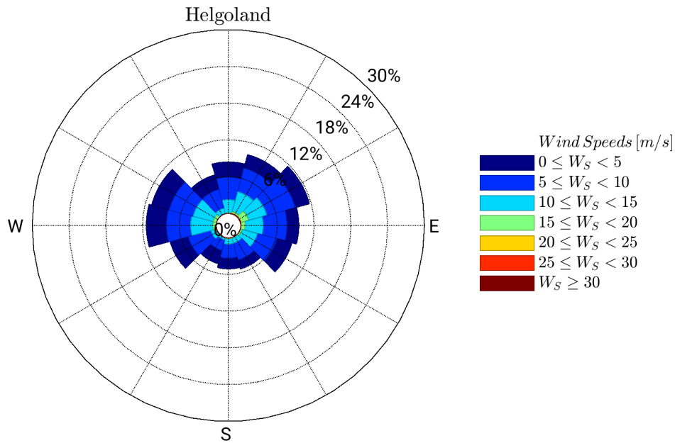
Abbildung 4: Windrose in Helgoland im Jahr 2002, Wind in Strömungsrichtung dargestellt.
