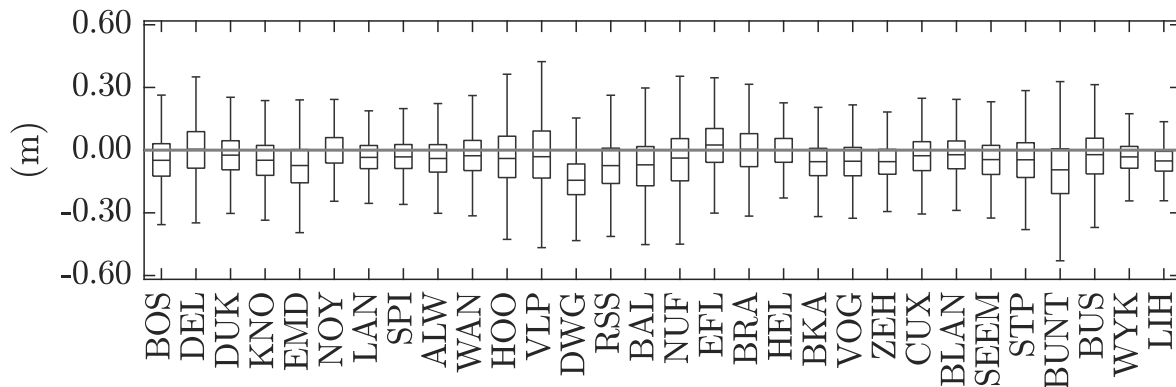
Abbildung 10: Fehlerverteilung des Wasserstandes im 2002
